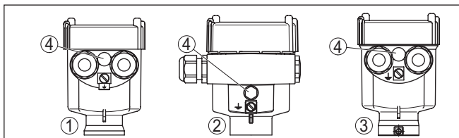
Fig. 10: Materiaalvarianten eenkamerbehuizing
