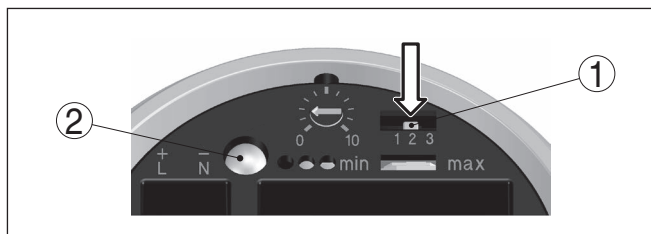
Fig. 16: Compensatieknop
